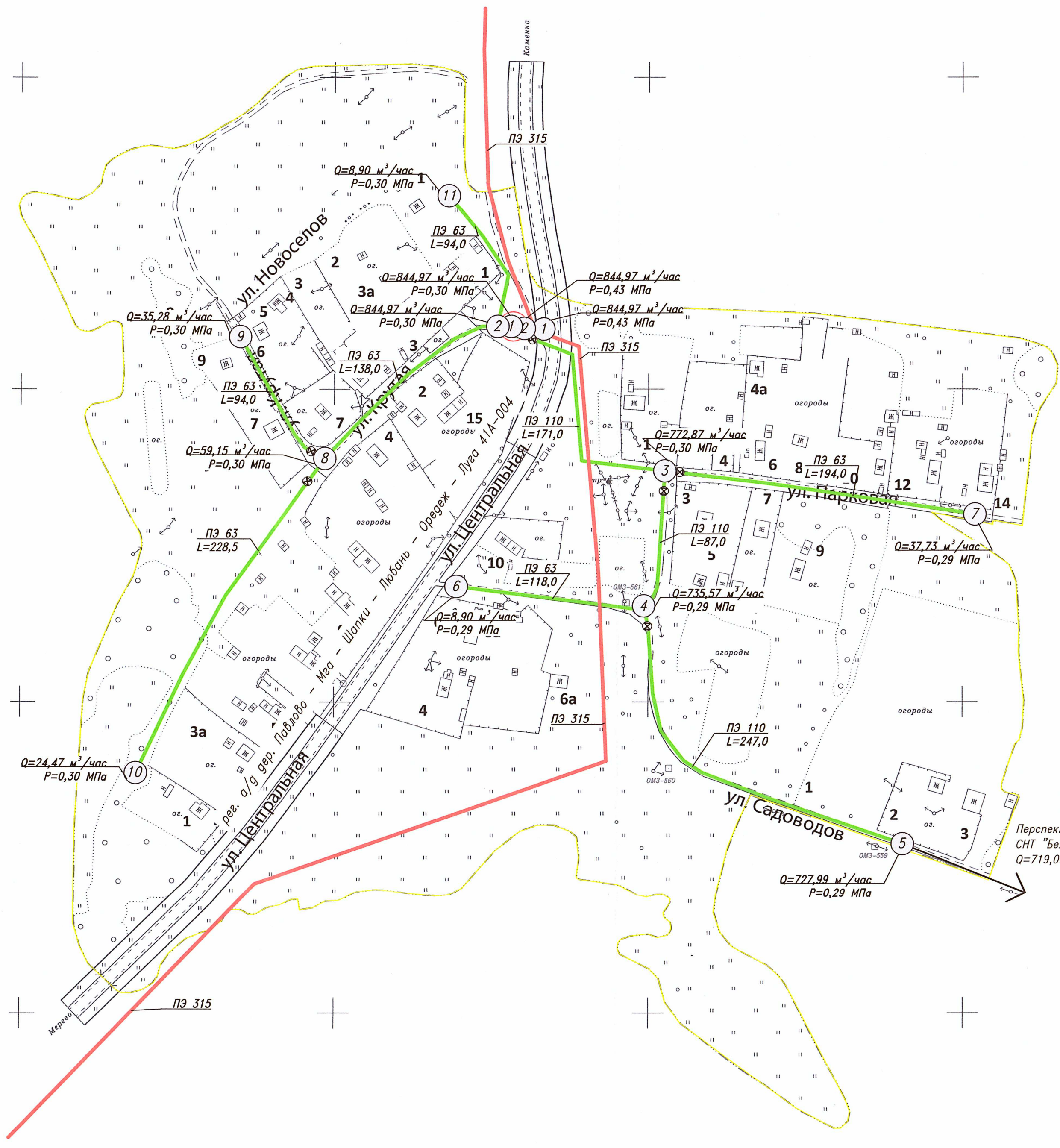
Гидравлический расчет газопровода высокого давления
